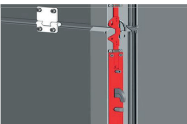
Serrure à crochets haute et basse
