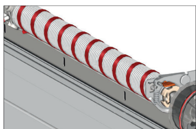
Ressorts de torsion traités par poudrage
