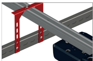
Motorisation et système easyfix
