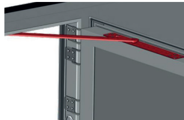
Ferme-porte encastré avec blocage à 90°
