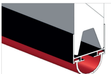
Joint à bulle EPDM sur panneau bas
