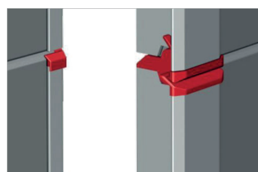
Embouts d'articulation sur dormant et ouvrant
