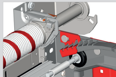
Renfort supérieur Renforcement de la courbe anti-dégondage
