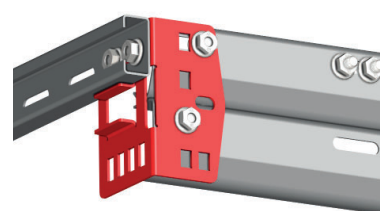
Equerre renforcée sur barre d'écartement
