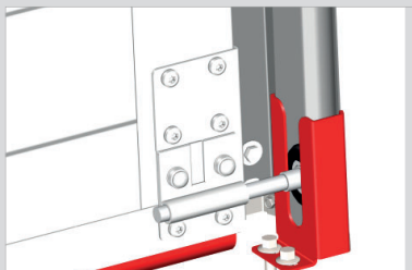
Sabot anti-effraction Sécurise le galet inférieur Fixé sur le rail vertical et au sol
