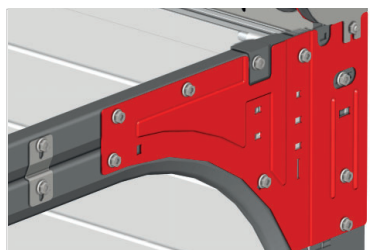
Renfort d'angle sur courbe de renvoi
