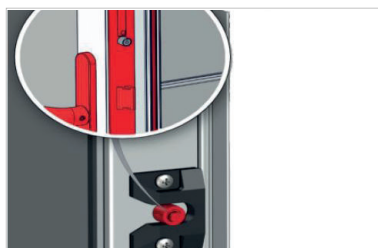
Doigts de centrage réglables par excentrique
